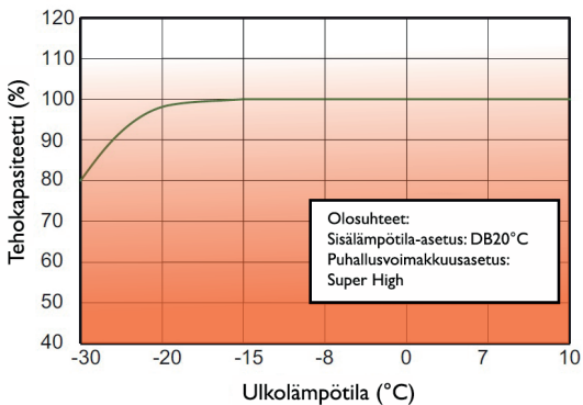
Lämmitysteho eri ulkolämpötiloissa
